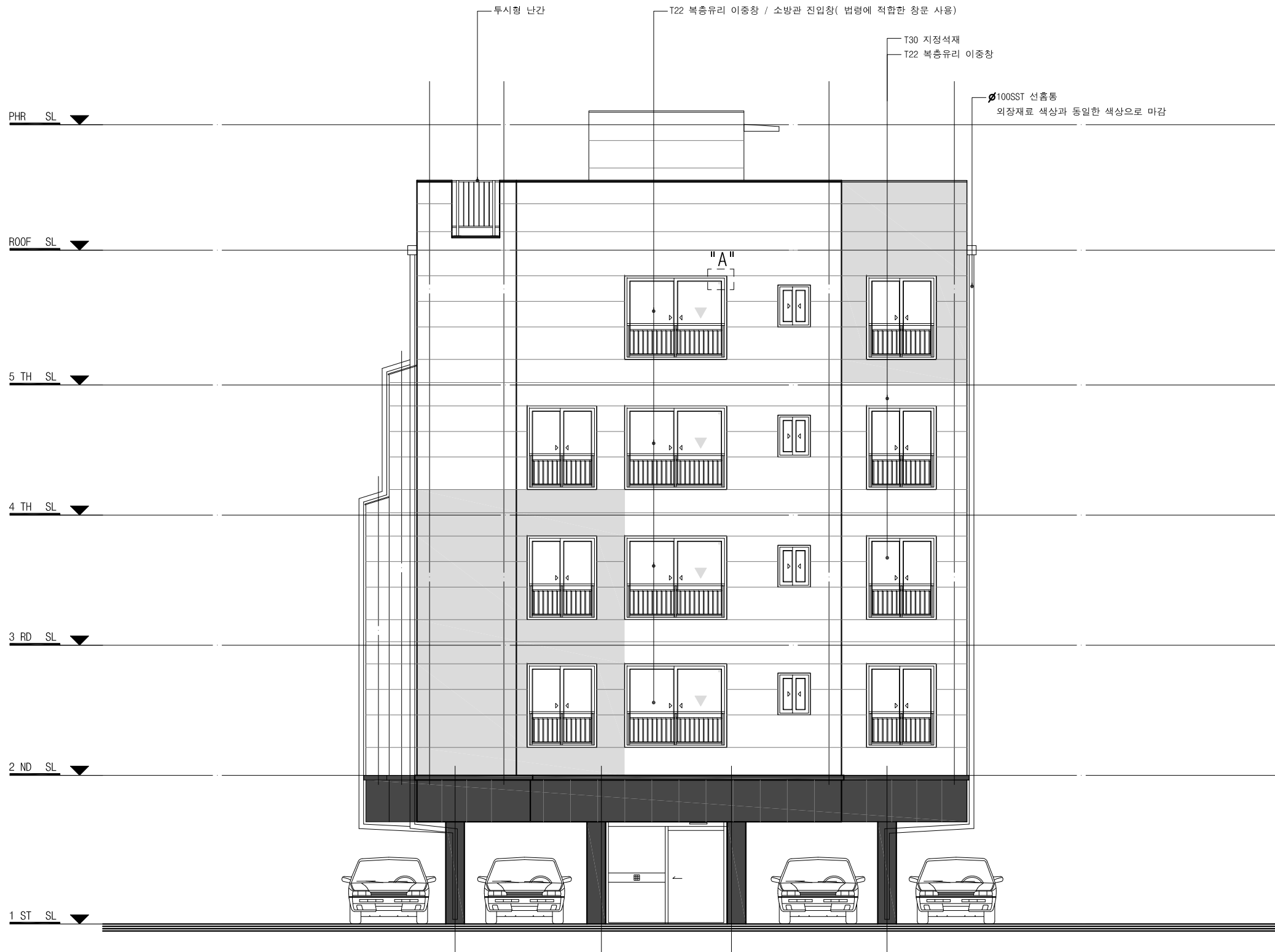
정 면 도 SCALE:1/100
