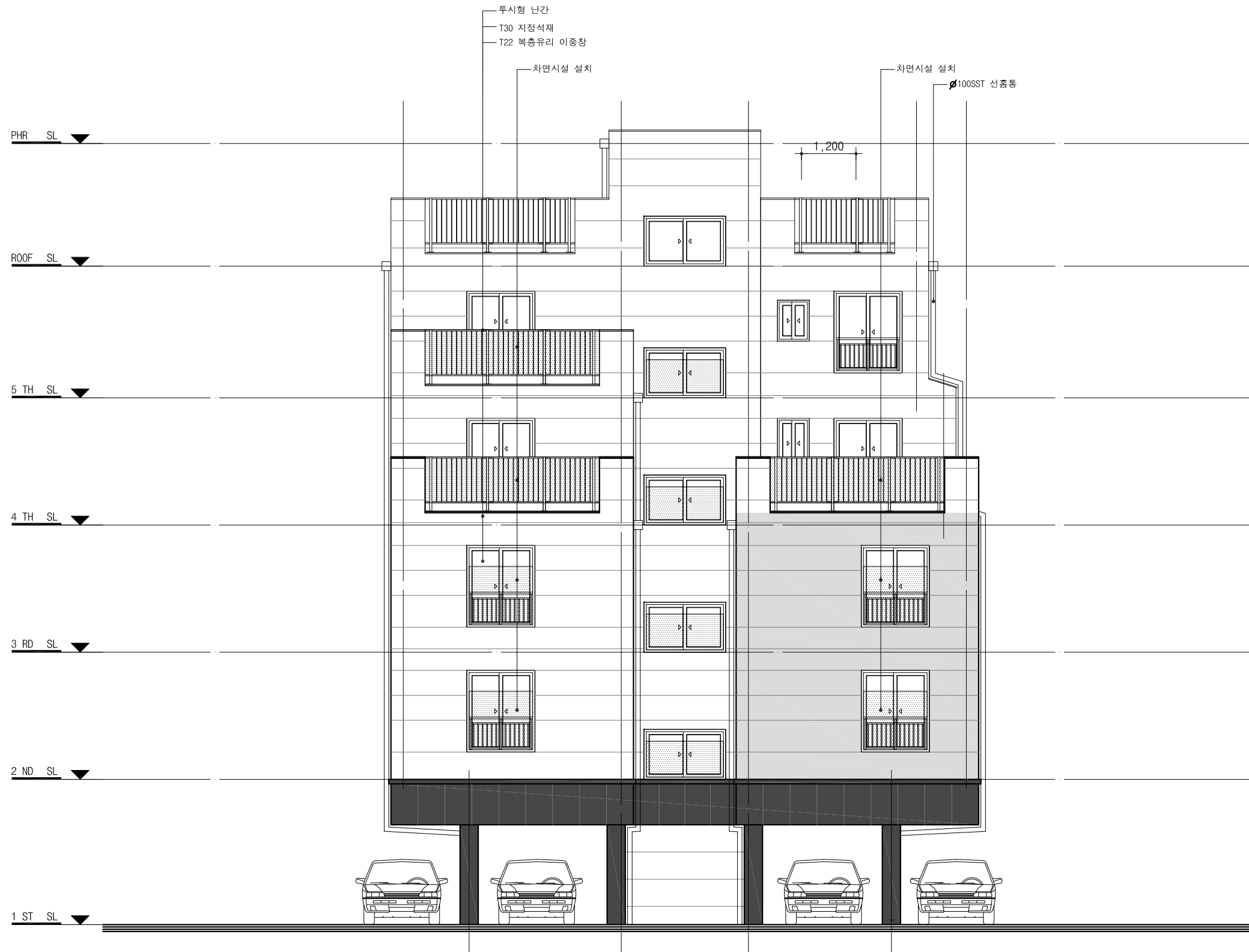
배 면 도 SCALE: 1/100
